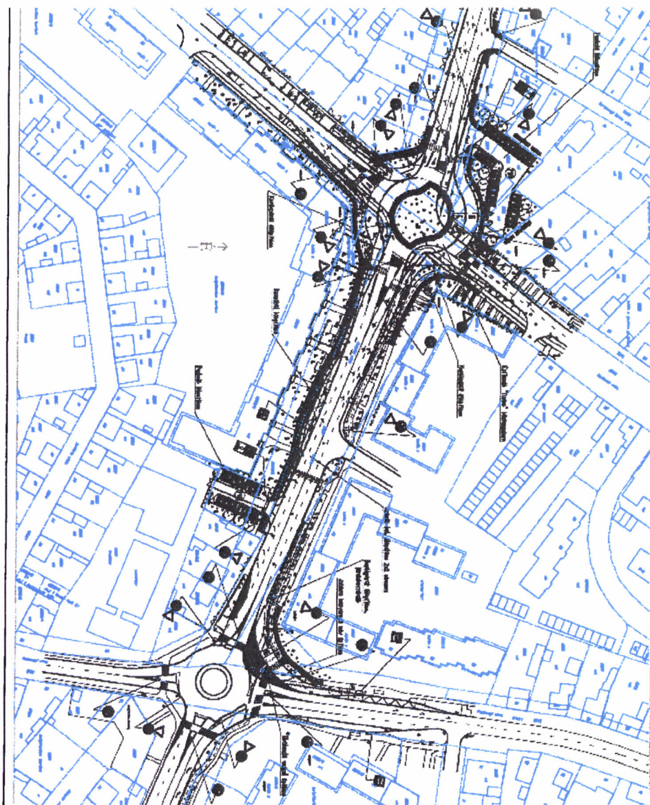
Forgalomtechnikai helyszínrajz
