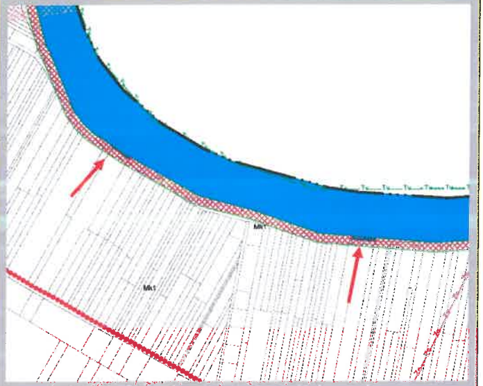
A 5. sz. terület javasolt módosítás szerinti szabályozási tervi részlete
